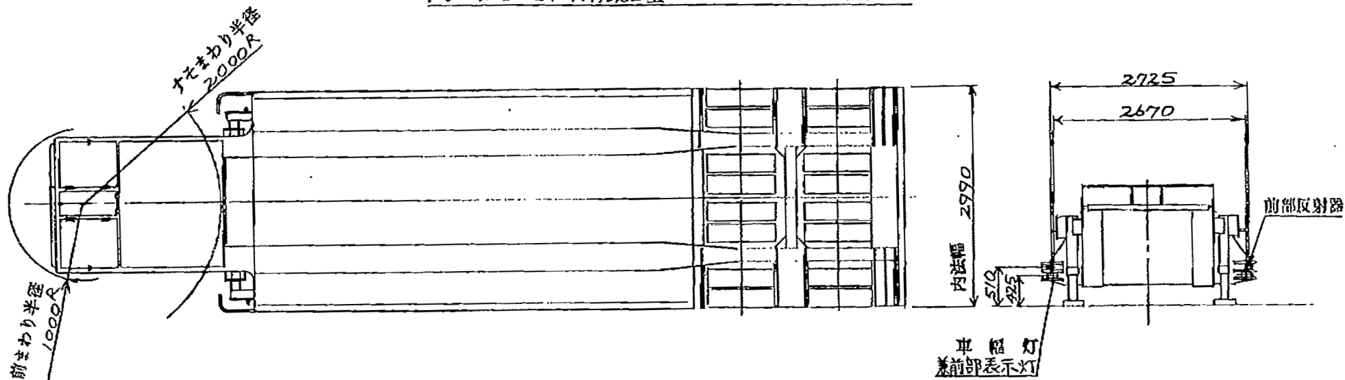
トールモービル PM439SL 型 セミトレーラ 外観四面図
